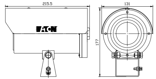
EACF-101Bカメラ
